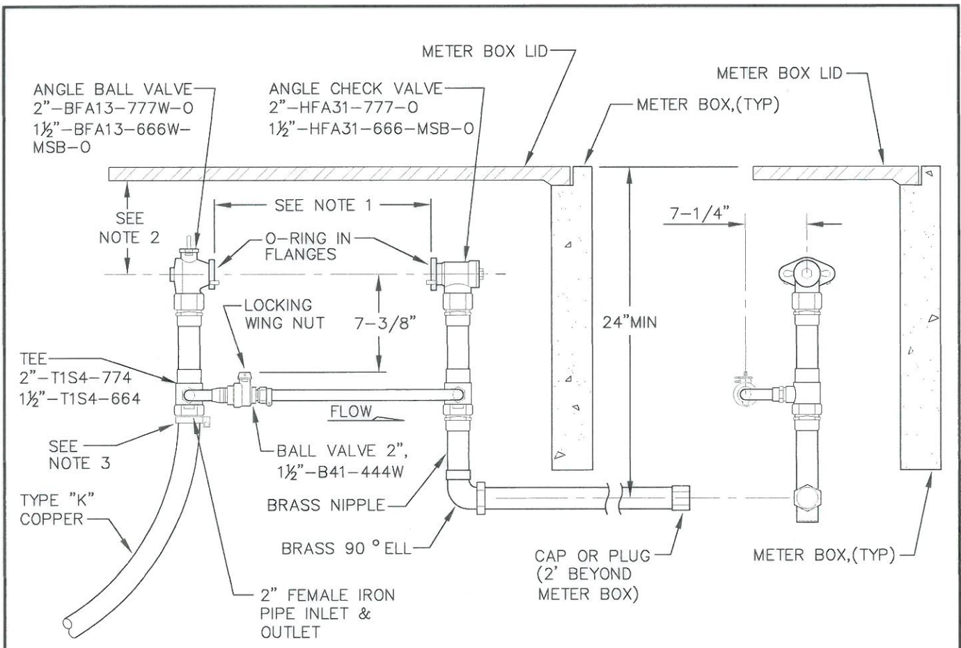
ELEVATION
