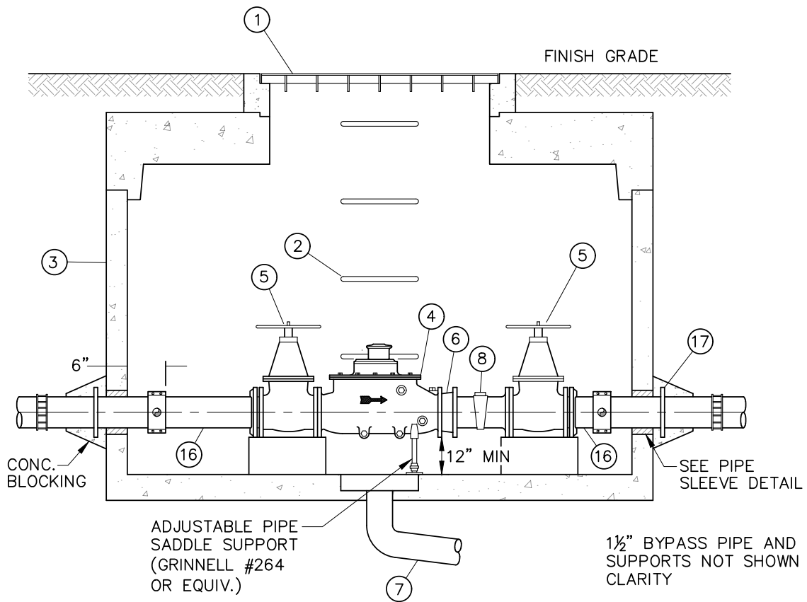
ELEVATION
